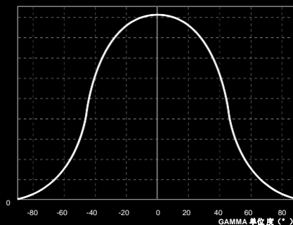
发光强度 (单位: CD/1000LM)
