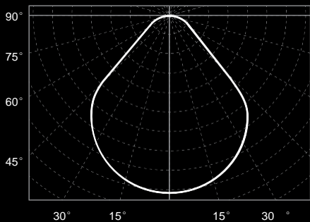
发光强度 (单位: CD/1000LM)
